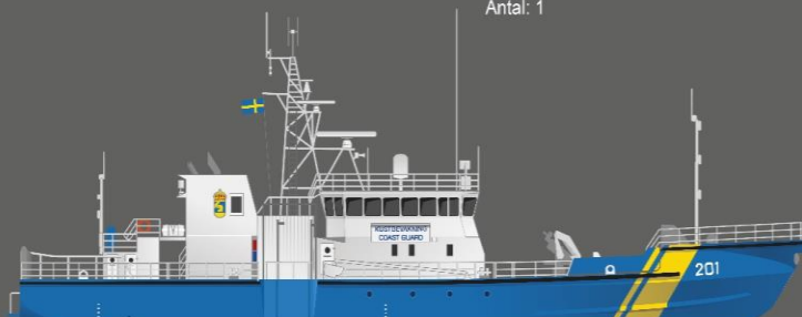
KBV 201-serien Längd: 52 m Bredd: 8,6 m Djupgående: 2,8 m Displacement: 476 ton Antal fartyg: 2
