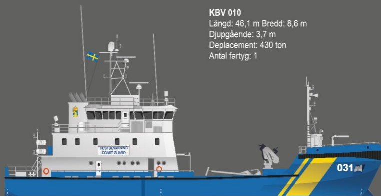
KBV 031-serien Längd: 51,1 m Bredd: 10,4 m Djupgående: 3 m Displacement: 948 ton Antal fartyg: 4
